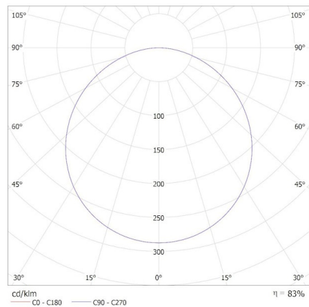
KANLUX S.A. (kat 37171) BLINGO 34W 4080 60NW / Krzywa rozsytu światła (biegunowo)
